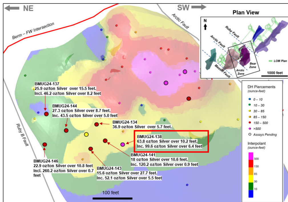
Long section looking SE (Azi 116-31)
